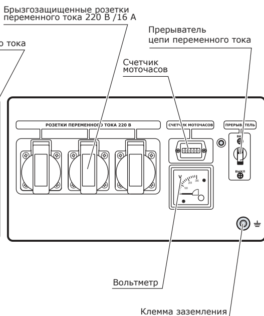
Рис. 10. Схема панели управления генератора УГД-5300 Basic
