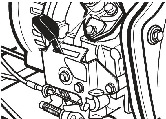
Рис. 18. Остановка генератора
