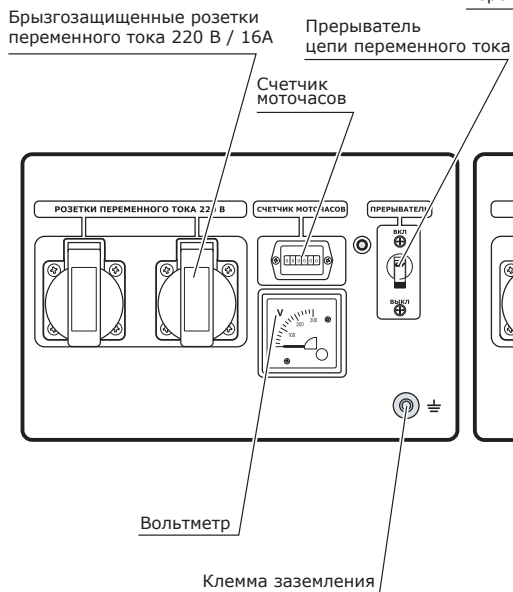
Рис. 9. Схема панели управления генераторов УГД-3000 Basic, УГД-4500 Basic
