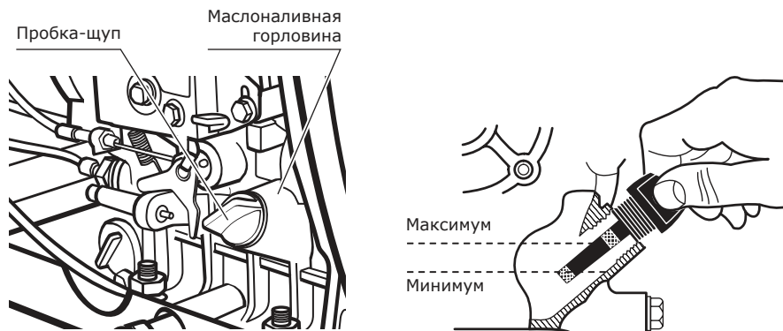
Рис. 11. Заполнение масляного картера и контроль уровня масла
